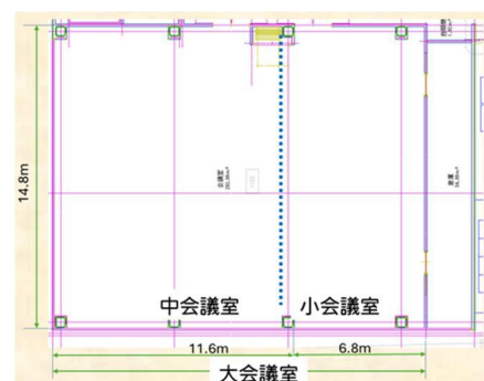
平面図
